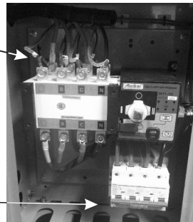
Mod.BFDE 40000
